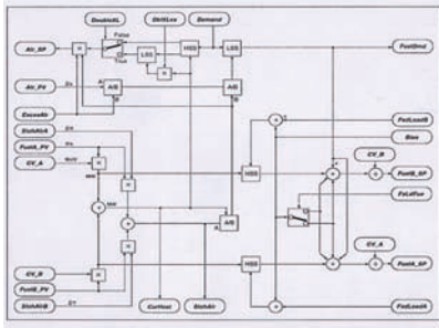
Schéma de principe du bloc MbnCtrl
